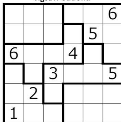
Jigsaw Sudoku
